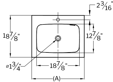
TOP VIEW / VUE DE DESSUS
